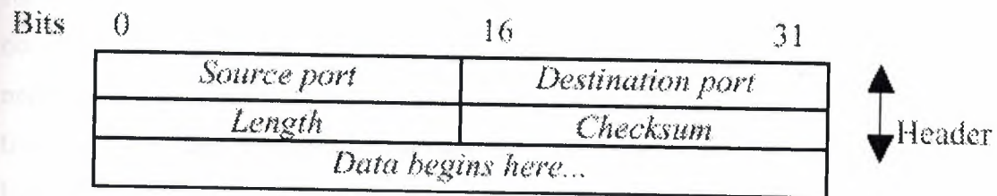
Figure 2.4. UDP Datagram
