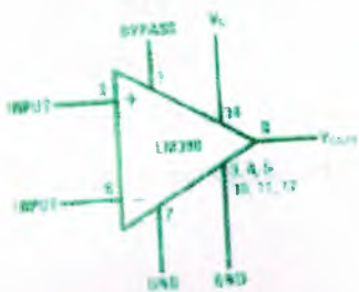
Fig.3.3 LM380N
