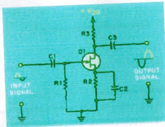
Fig. 2.3 FET audio amplifier
