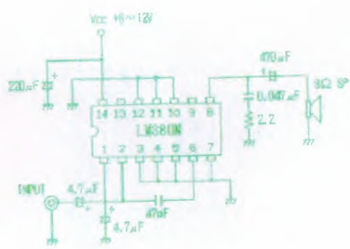
Fig. 4.3 LM380N
