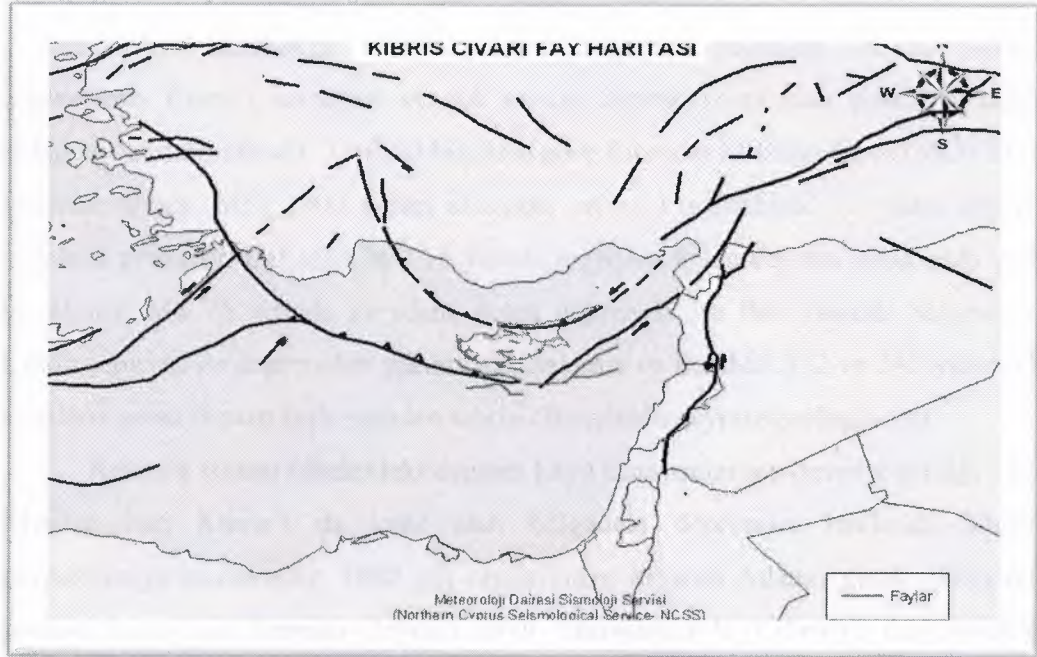
Şekil 2. Kıbrıs civarı fay hatları (MDM, 2010).
