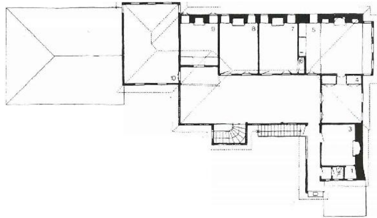
Şekil 5. 141 Hasan Bey Evi'nin planı (Bektaş, C. , 1996).
