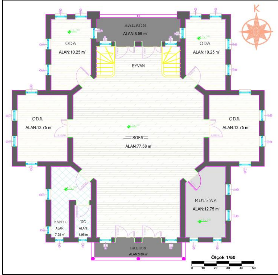
Şekil 5. 146 Aksaray İli'nin Merkez İlçesi'nde bulunan Çorakçılar Konağı'nın birinci kat planı (Bediha Uğur).
