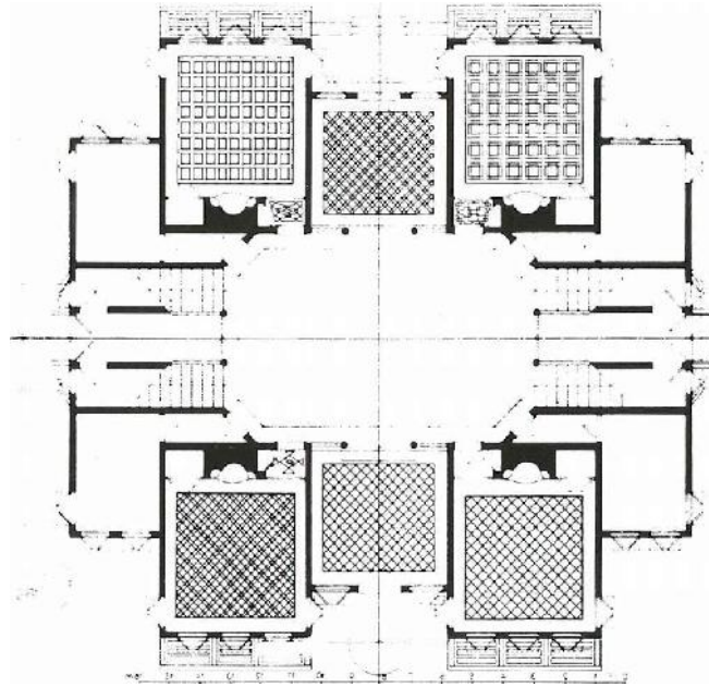
Şekil 5. 145 Çengelköy, Sadullah Paşa Yalısı'nın planı (18.yy. Sedat Hakkı Eldem. Türk Evi ,Taç Yayınları kitabından alınmıştır) (Bektaş, C. , 1996).
