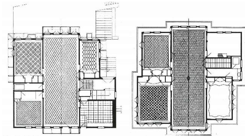
Şekil 5. 143 Hasköy, Hahambaşı Konağı’nın planı (18.yy. Sedat Hakkı Eldem. Türk Evi ,Taç Yayınları kitabından alınmıştır) (Bektaş, C. , 1996).
