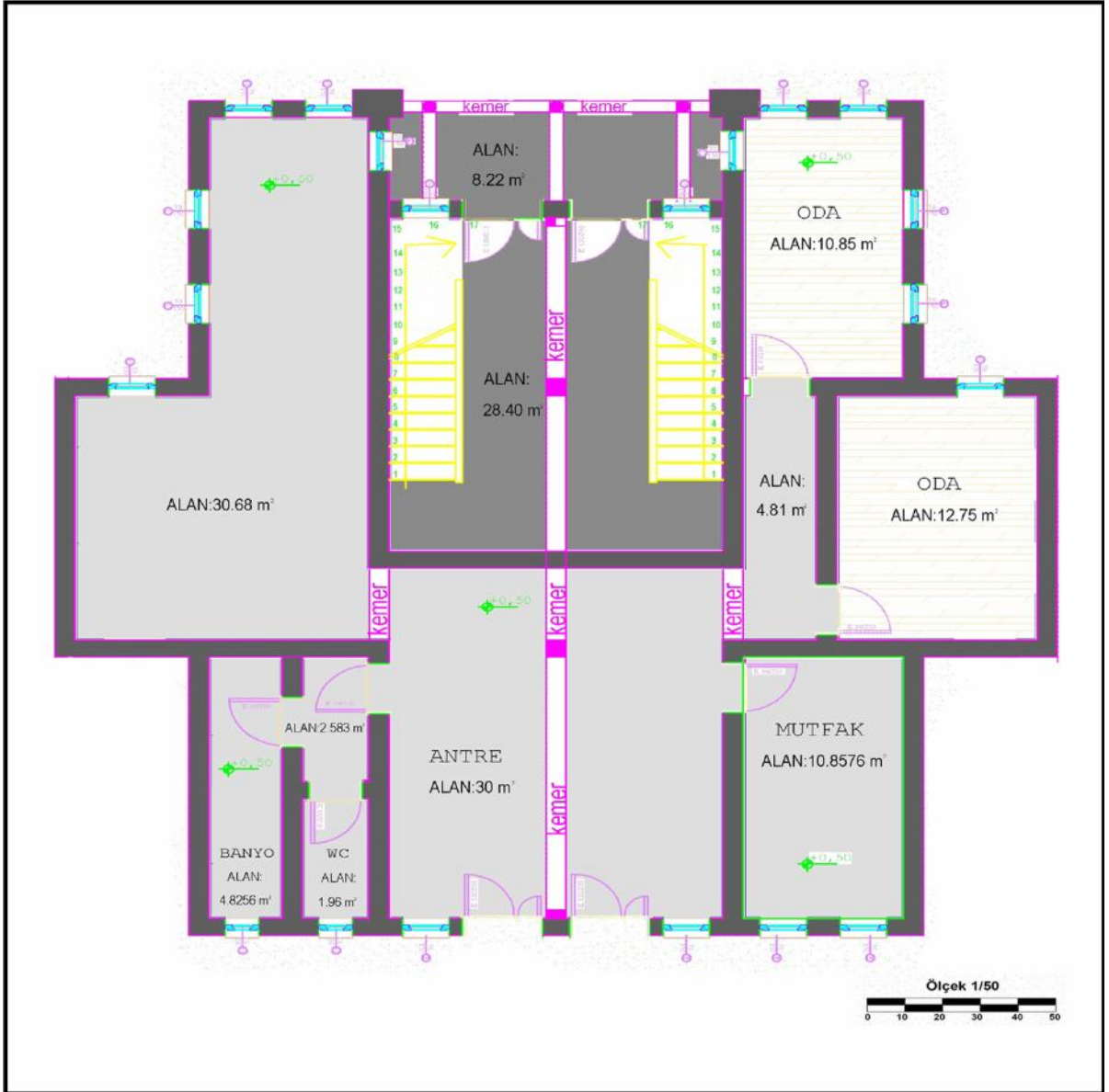
Şekil 5. 90 Çorakçılar Konağı'nın zemin kat planı (Bediha Uğur).
