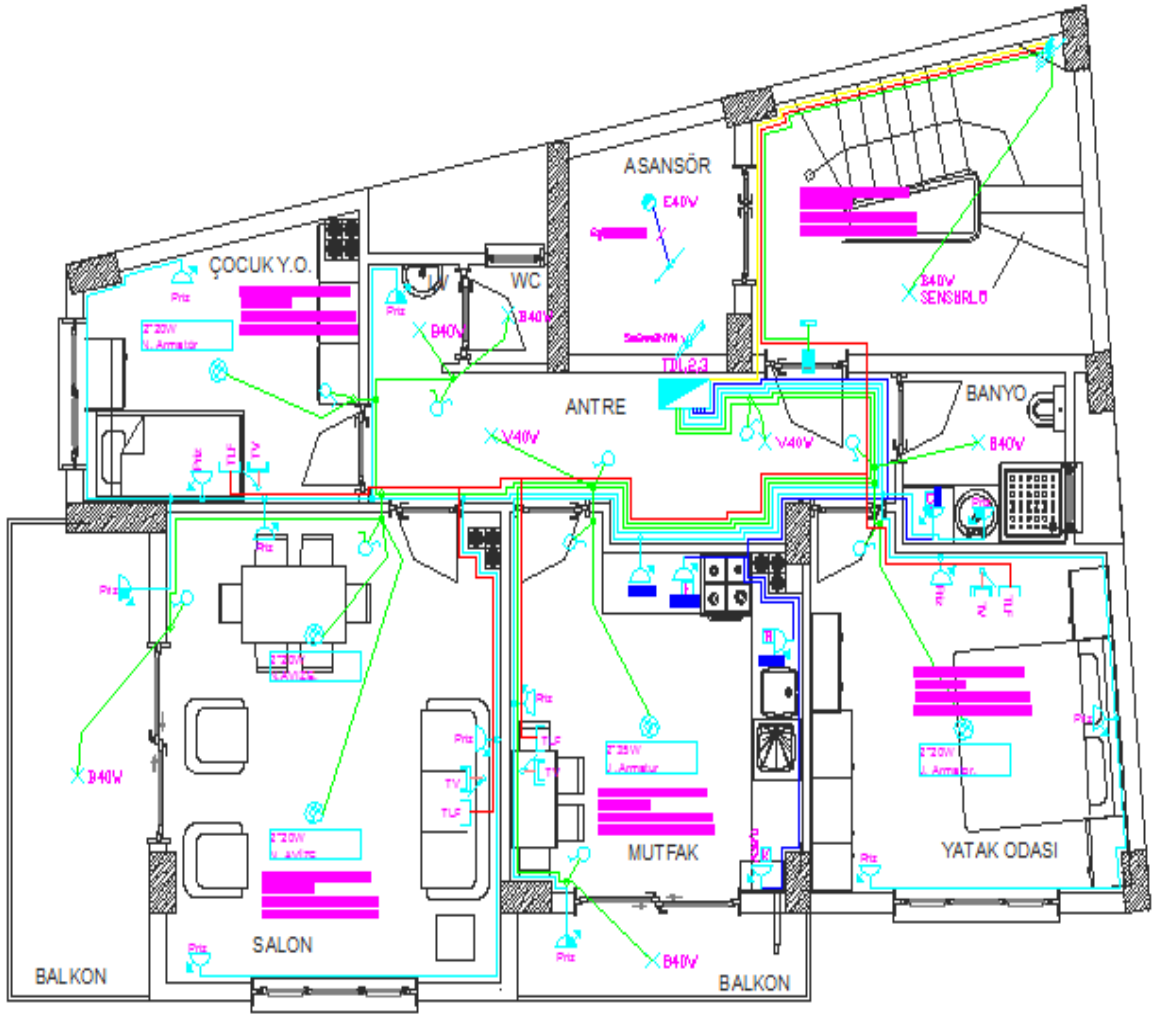
Şekil 1.1: Aydınlatma, priz, zayıf akım sembolleri.
