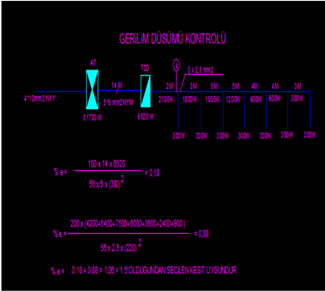
Şekil 3.1: Gerilim düşümü hesabı
