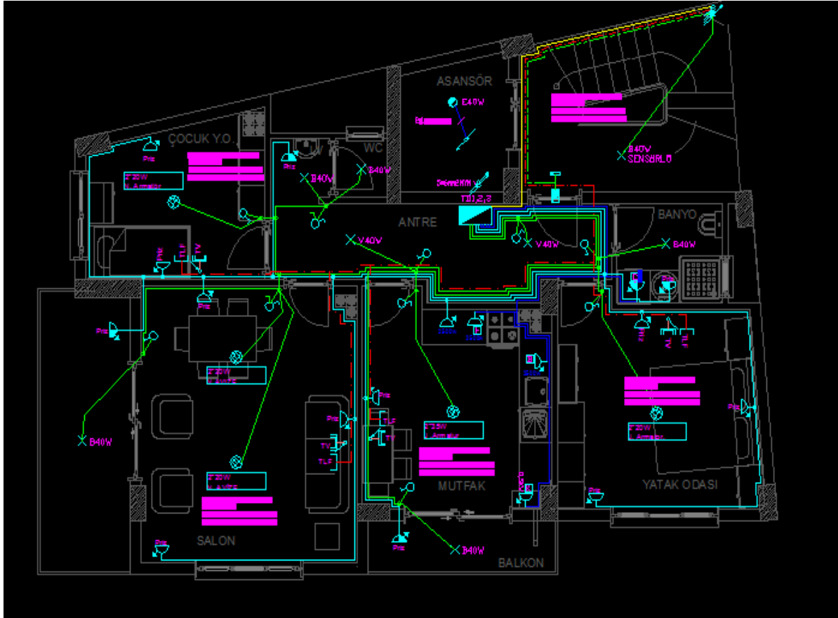
Şekil 1.4: priz, armatür çizim
