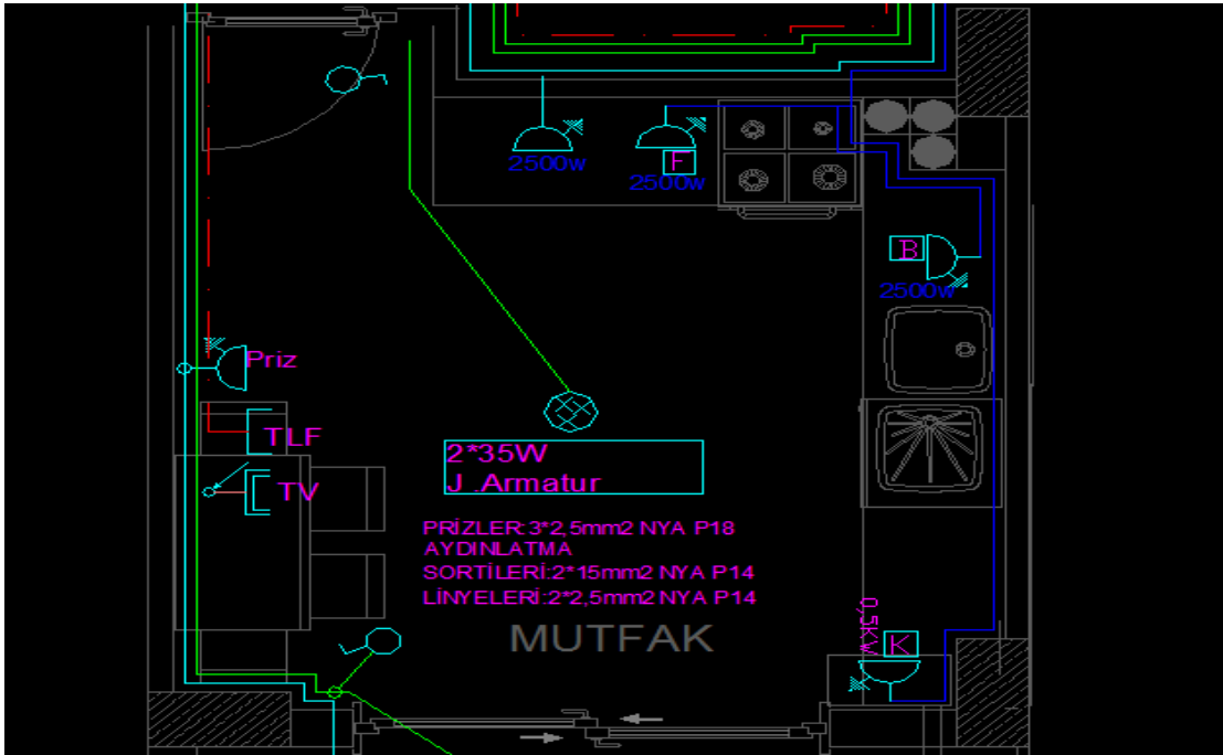
Şekil 1.7: Aydınlatma sortisi çizimi.
