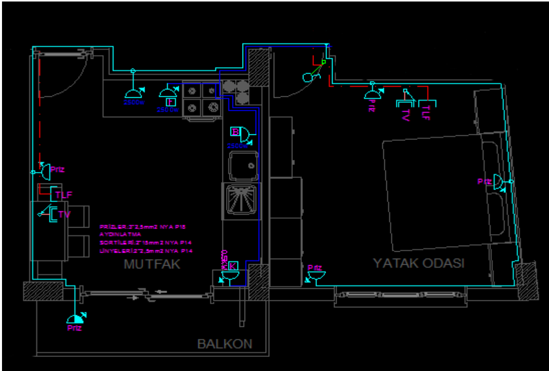
Şekil 1.9: Telefon tesisi.
