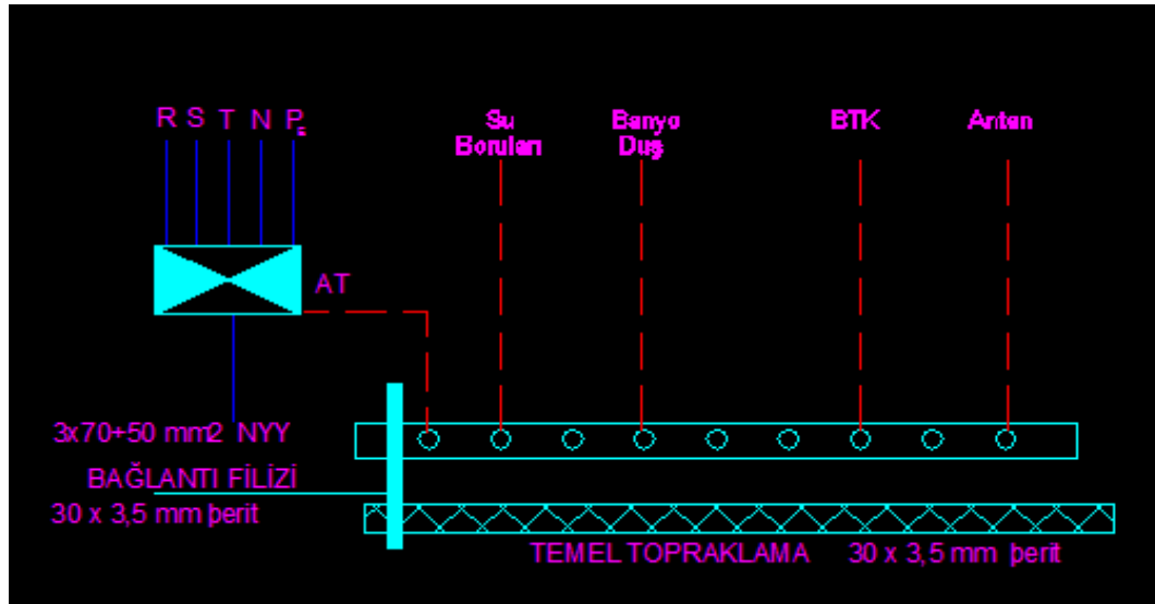
Şekil 3-3: temel topraklaması
