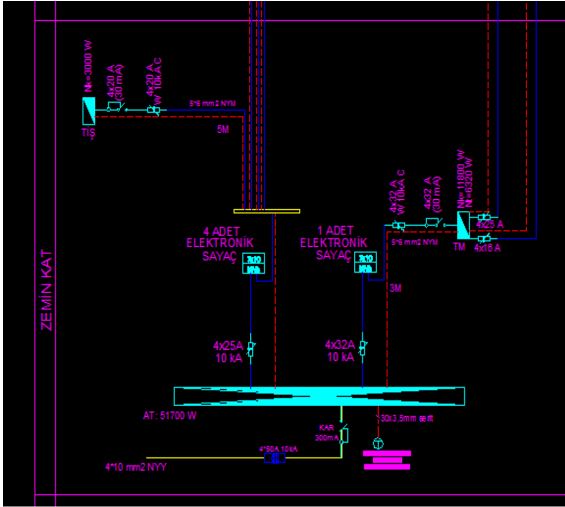
Şekil 2.1: Kolon Şeması.
