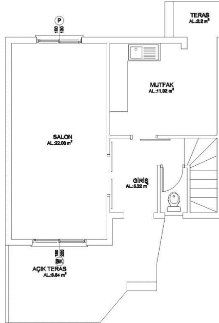
Şekil 4.3: Göçmenköy Sosyal Konutları Zemin Kat Planı (İnançoğlu, 2018)
