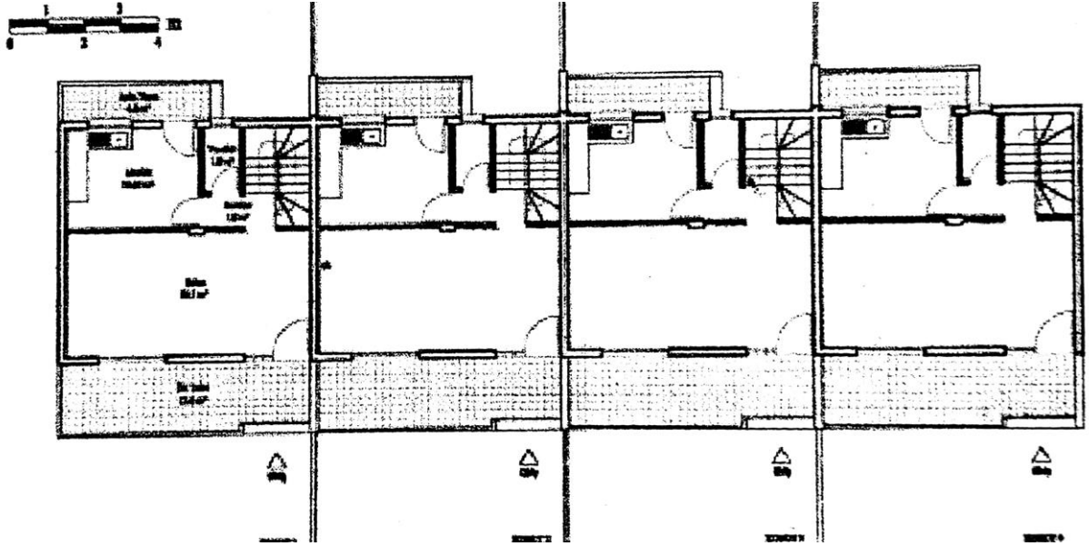
Şekil 3.16: Devlet Sosyal konutlarının zemin kat planı lineer tip (Sarıyer, 2001 ).
