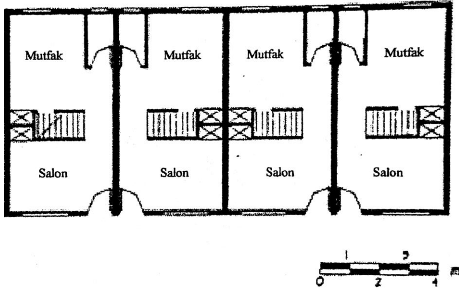
Şekil 3.13: Göçmen evi dörtlü sıra, zemin kat planı (Keleş, 1998).
