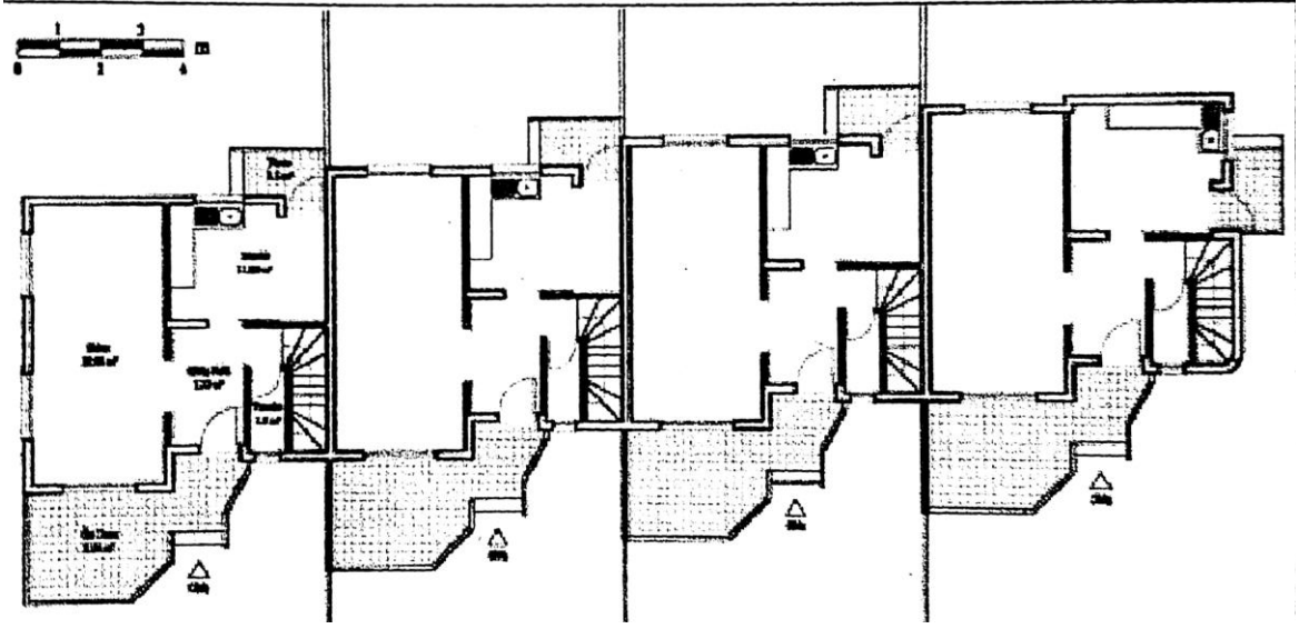
Şekil 3.15: Devlet Sosyal konutlarının zemin kat planı zigzag tipi (Sarıyer, 2001 ).
