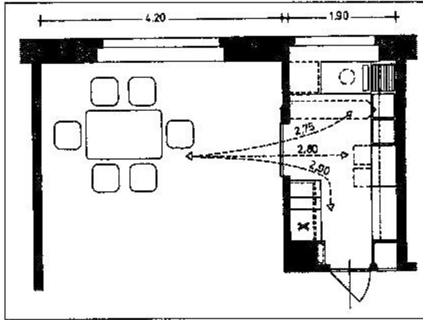
Şekil 2.3: Frankfurt mutfak planı ve yemek odası ile bağlantısı (Kürüm, 2009)
