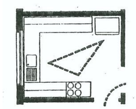
Şekil 2.14: U tipi mutfak planı (Arcan-Evci, 1992)
