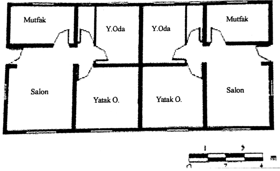
Şekil 3.12: Göçmen evi planı, iki yatak odalı tip-2 (Keleş, 1998).
