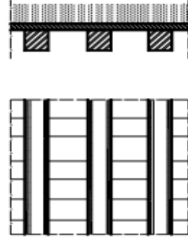
Şekil 3.18: Ters tavan kesit ve detayı (Uludağ, 2017)
