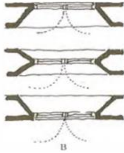
(b) Kalın duvarın inceltilmesi
