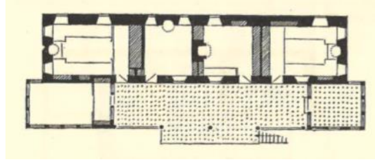
Şekil 2.3: Dış sofalı plan tipi (Eldem, 1954)
