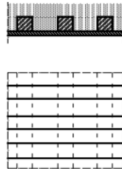
Şekil 3.20: Düz tavan detayı (Yıldırım ve Hidayetoğlu, 2006)
