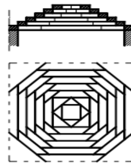
Şekil 3.23: Kırlangıç Tavan detayı (Uludağ, 2017)
